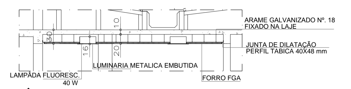
CORTE F-F ESCALA:.....1/50 SANCA DE ILUMINAÇÃO SL. DE ESPERA / RECEPCAO / CIRCULACAO
