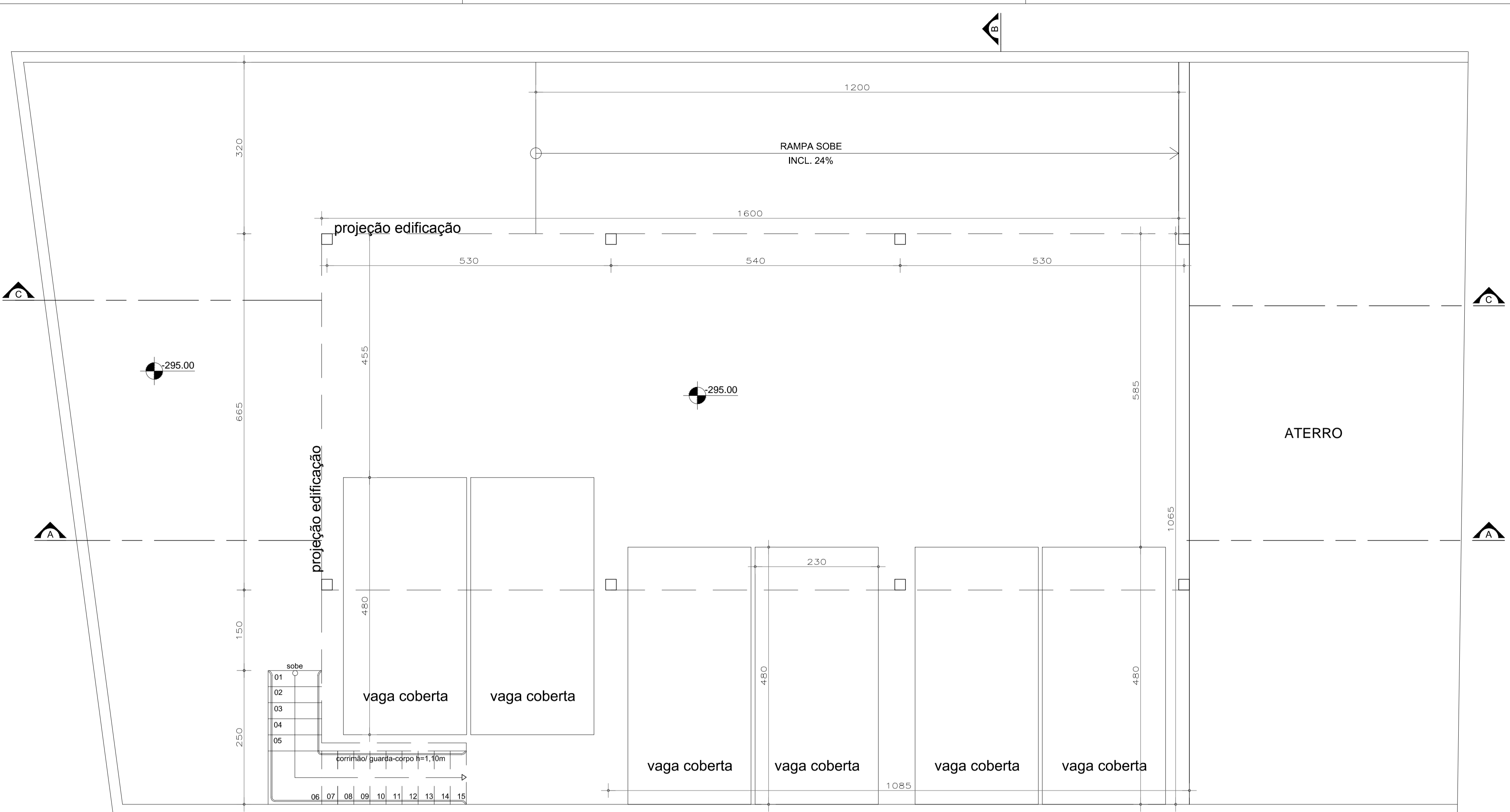
PLANTA BAIXA - SUBSOLO ESCALA:.....1/50 ÁREA = 107,8 m² INDICA O INÍCIO E SENTIDO DA PAGINAÇÃO
